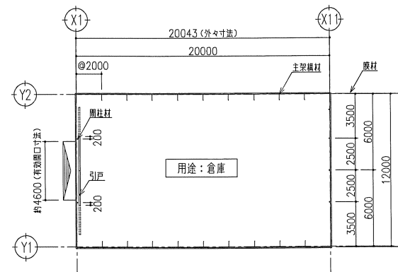
平面図 S=1/200
