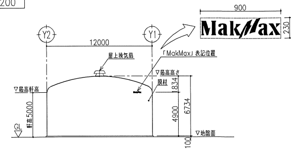
立面図 S=1/200 (X11通り)
