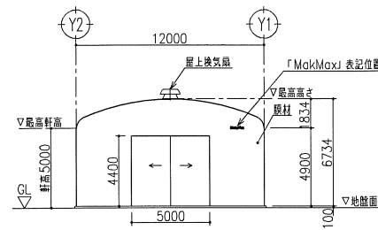
立面図 S=1/200 (X1通り)
