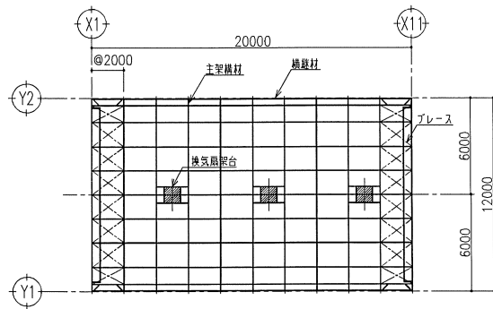
小屋伏図 S=1/200
