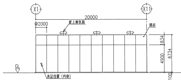
立面図 S=1/200 (Y1, Y2通り)
