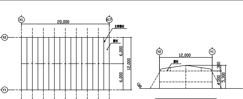
屋根伏図 S=1/200
