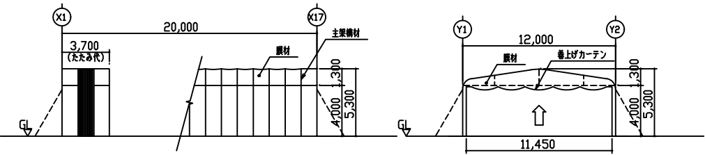
側面図 S=1/200 (Y1通り)
