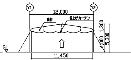
正面図 S=1/200 (X17通り)
