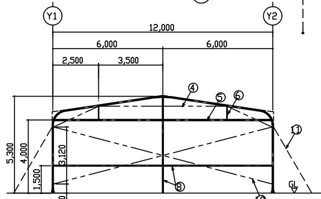
軸組図 s=1/100 (X1, X17通り)
