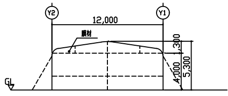
立面図 S=1/200 (X1通り)
