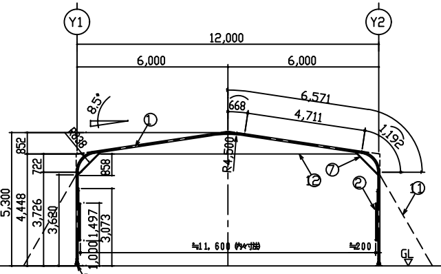
断面図 s=1/100 (X2~X16通り)
