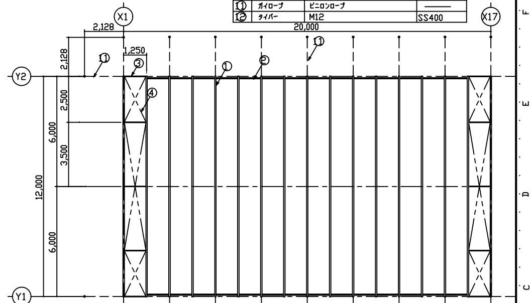
小屋伏図 s=1/100
