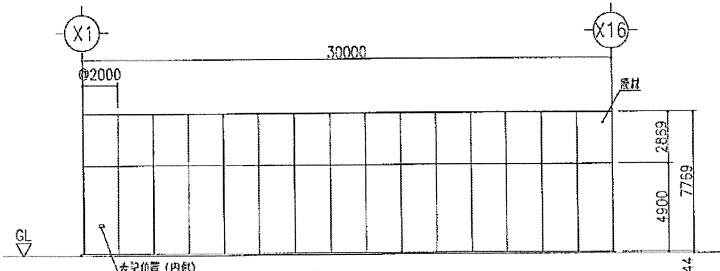
立面図 S=1/200 (Y1, Y2通り)
