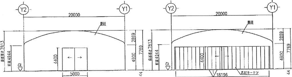
立面図 S=1/200 (X1, X16通り)
