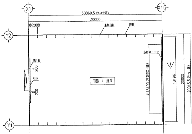
平面図 S=1/200
