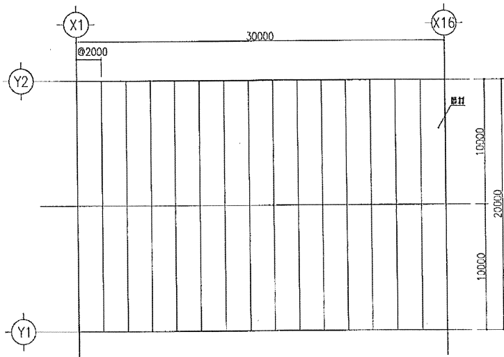
屋根伏図 S=1/200
