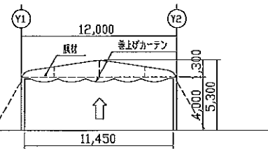
正面図 S=1/200 (X17通り)
