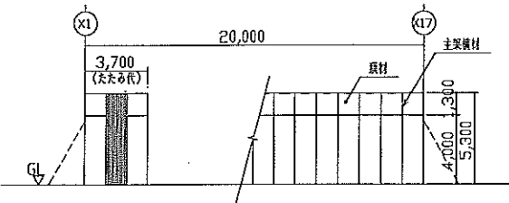
側面図 S=1/200 (Y1通り)
