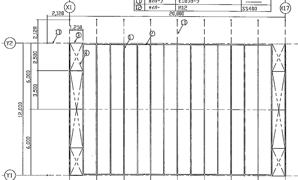
小屋根伏図 s=1/100
