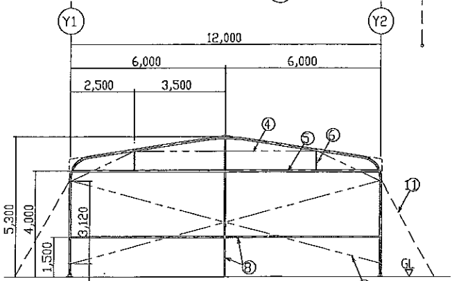
輪組図 s=1/100 (X1, X17通り)
