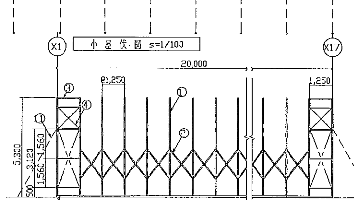
輪組図 s=1/100 (Y通り)
